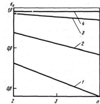
Рисунок 11 – Графики K = f(n) при P_1 = P_2 = P_3 = P_i = \lambda ; v = 30\% для r = 0 (1); 1 (2); 5 (3); \infty (4)
