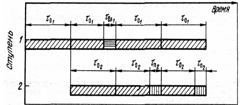
Рисунок 4 – График протекания производственного процесса в двухфазной системе с жесткой связью
