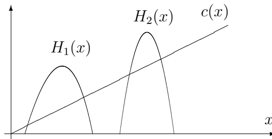
Рис. 3. Определение множества возможных равновесий
