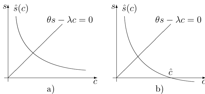
Рис. 5. Различные варианты поведения функции \hat{s}(c) на фазовой плоскости.
