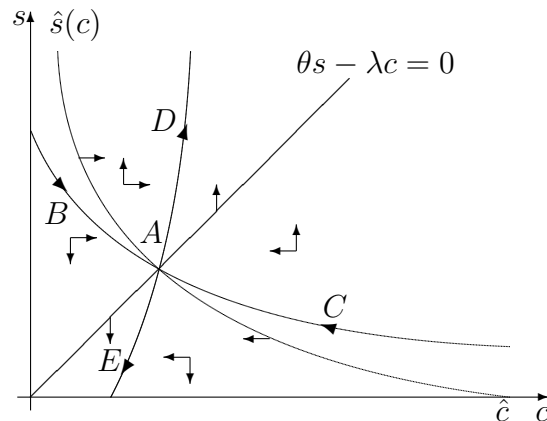
Рис. 6. Поле направлений для системы (142).
